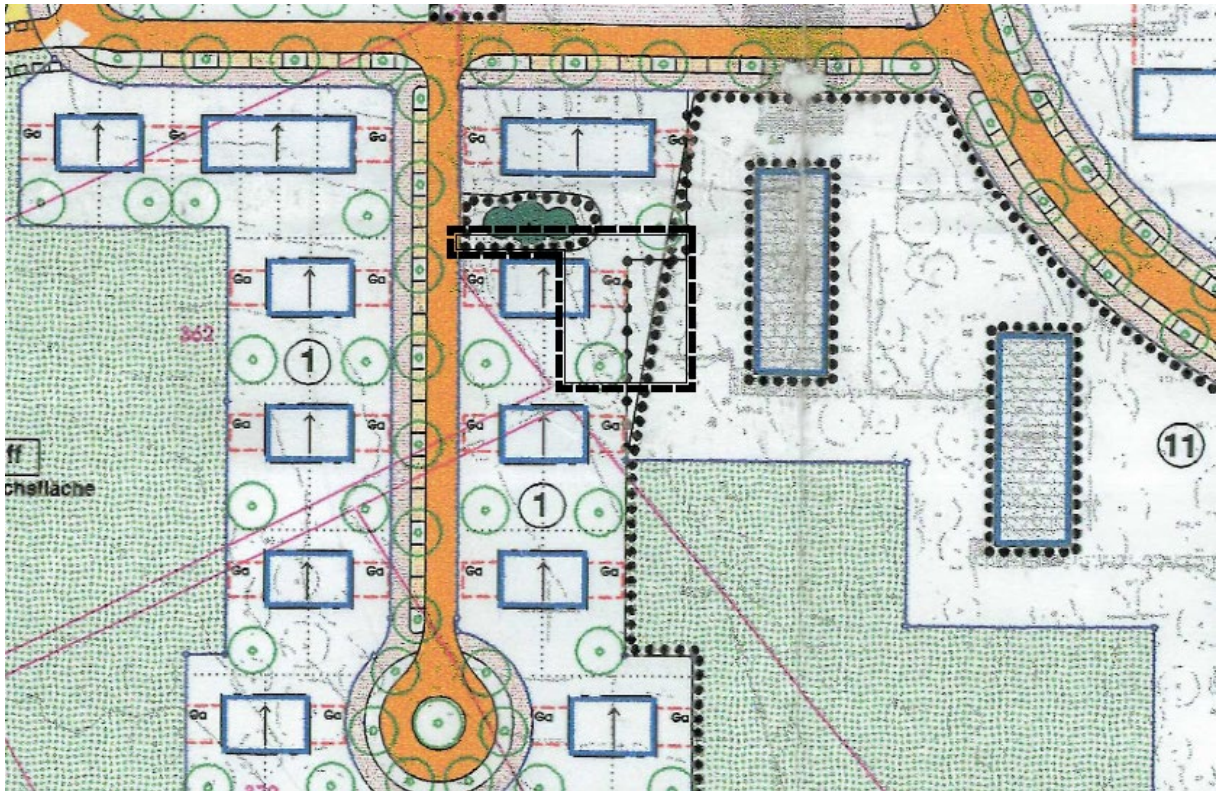
Ausschnitt Bebauungsplan „Solpark“ mit überlagertem Geltungsbereich der 24. Änderung, unmaßstäblich
