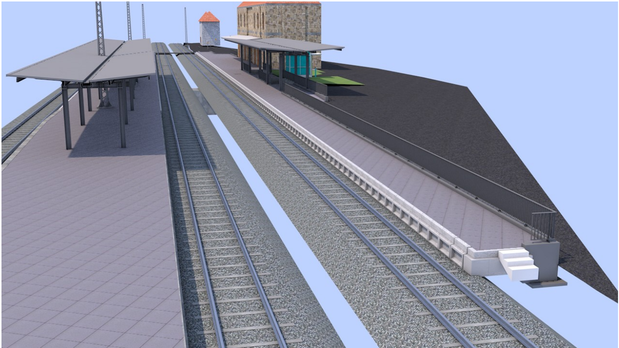
Vogelperspektive Gleis 1-3 (Geländer an Gleis 1 nachrichtlich, wird durch Anschluss Busbahnhof nicht erforderlich)
