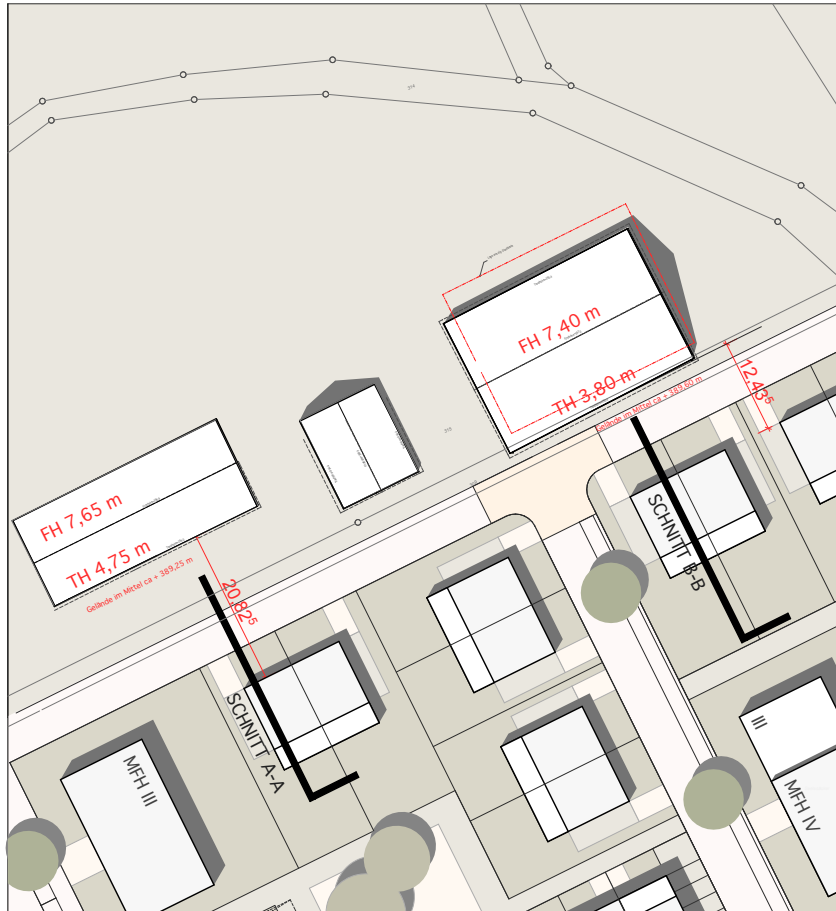
Lageplanausschnitt 1:1000
