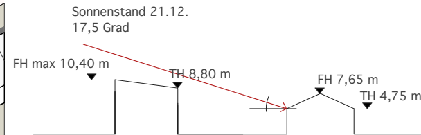
Bebauungsvariante mit Satteldach
