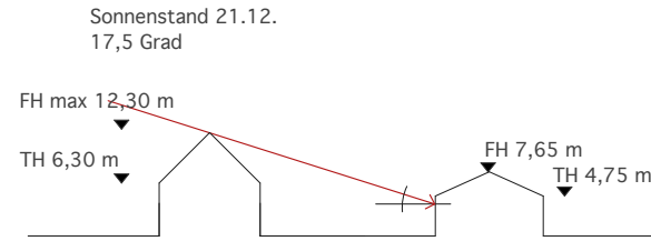
Bebauungsvariante mit Satteldach
