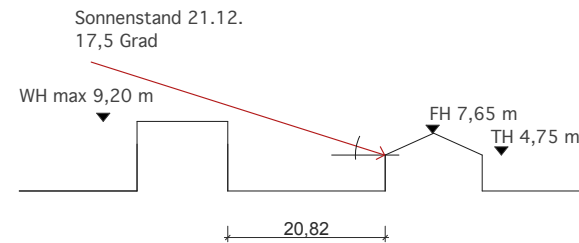
Bebauungsvariante mit Flachdach
