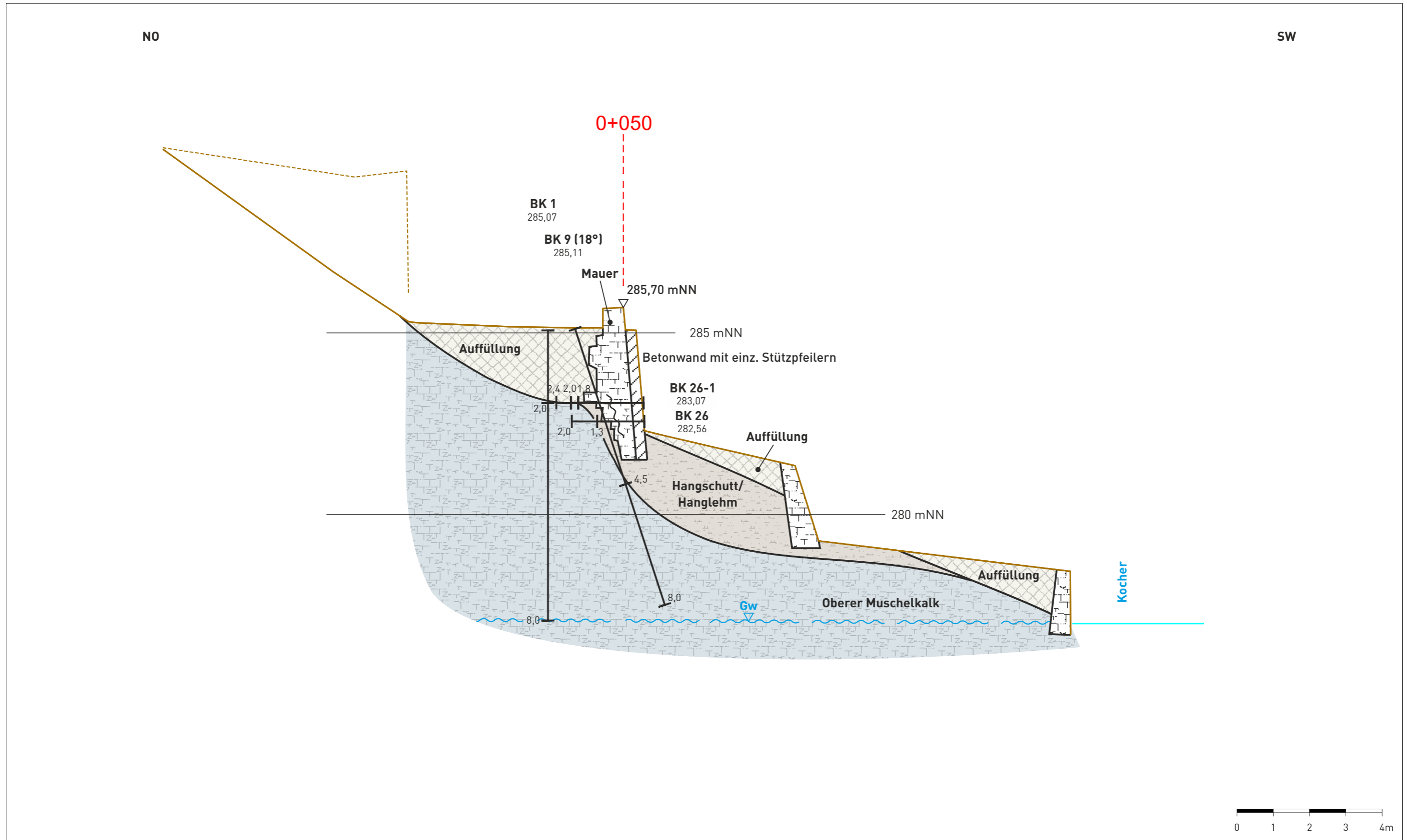
Geologischer NO-SW-Geländeschnitt 1 (0+050) (Schnittführung siehe Anlage 1.2.1)
