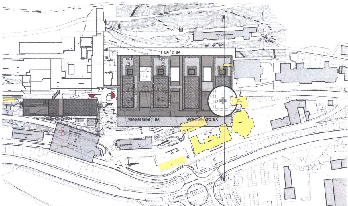
Lageplan 1. + 2.BA
