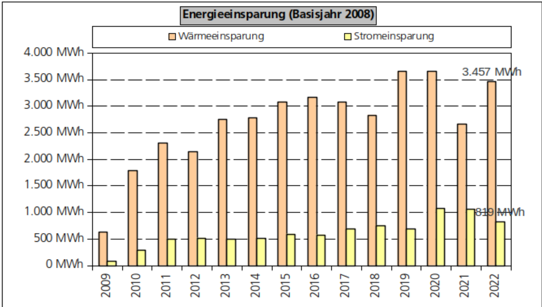
Diagramm 2 Energieeinsparung (Basisjahr 2008)
