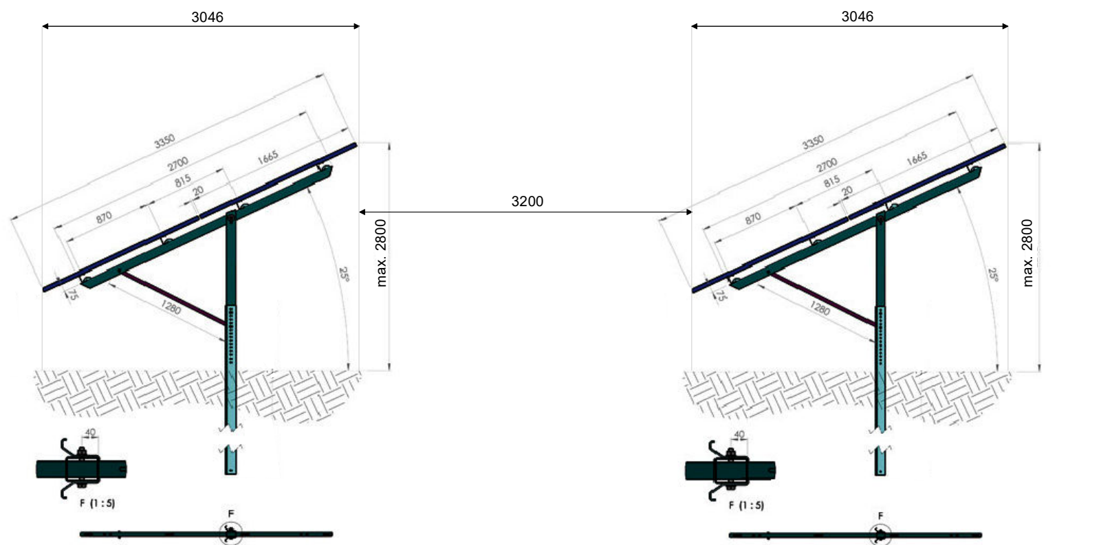
Schema der Modulaufstellung (M 1 : 50)
