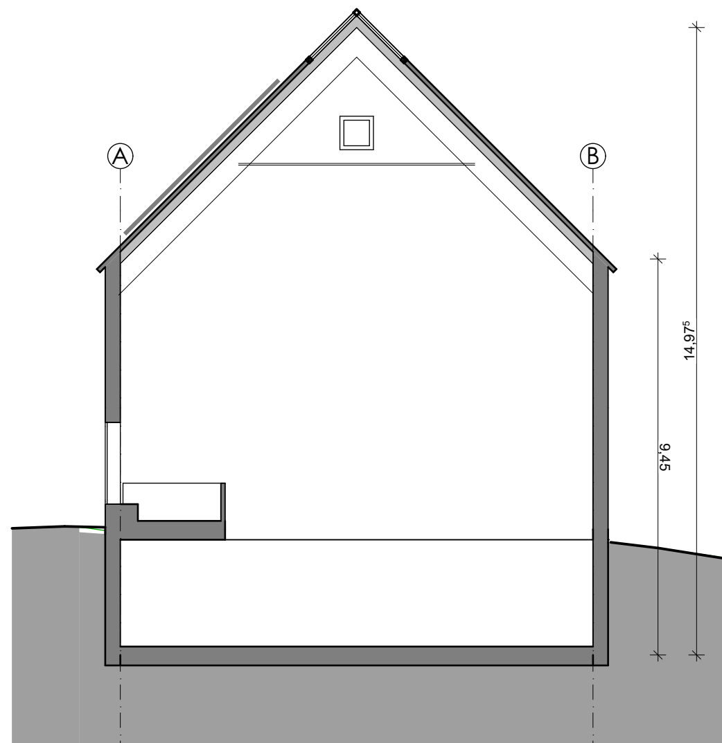
SCHNITT 1-1 - Kletterhalle
