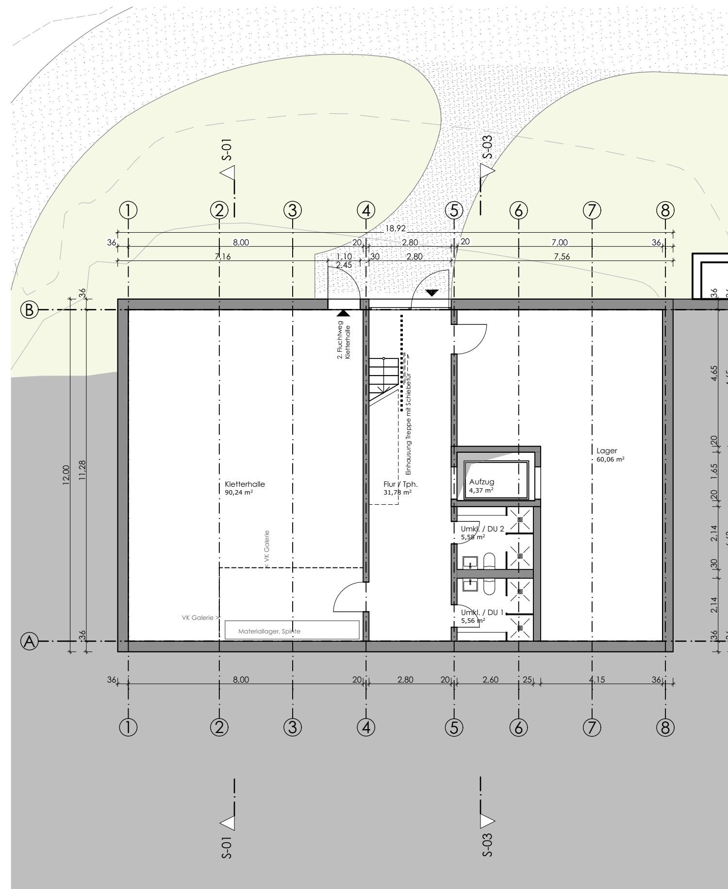
UNTERGESCHOSS (Teilunterkellerung)
