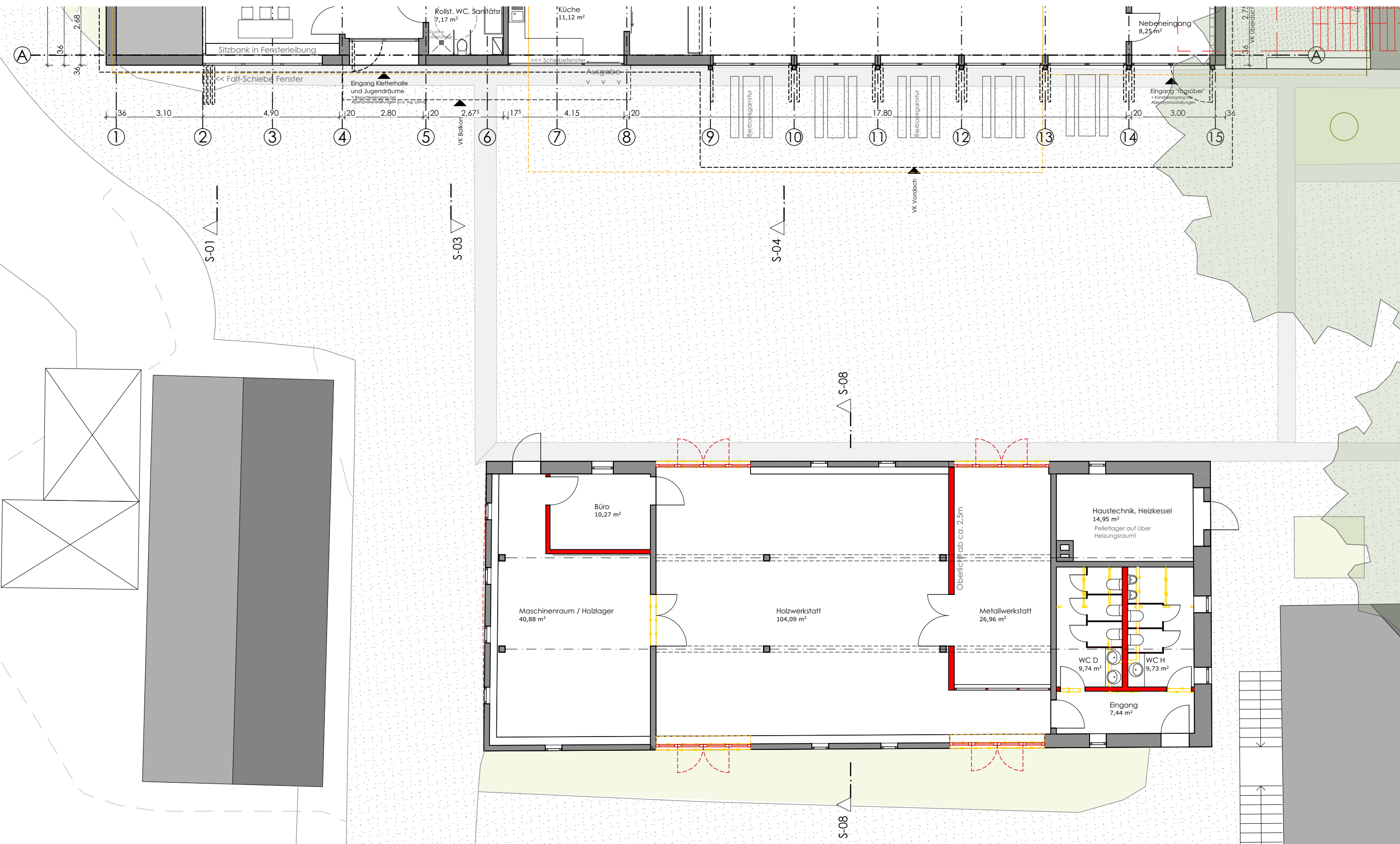
ERDGESCHOSS - Umbau Scheune
