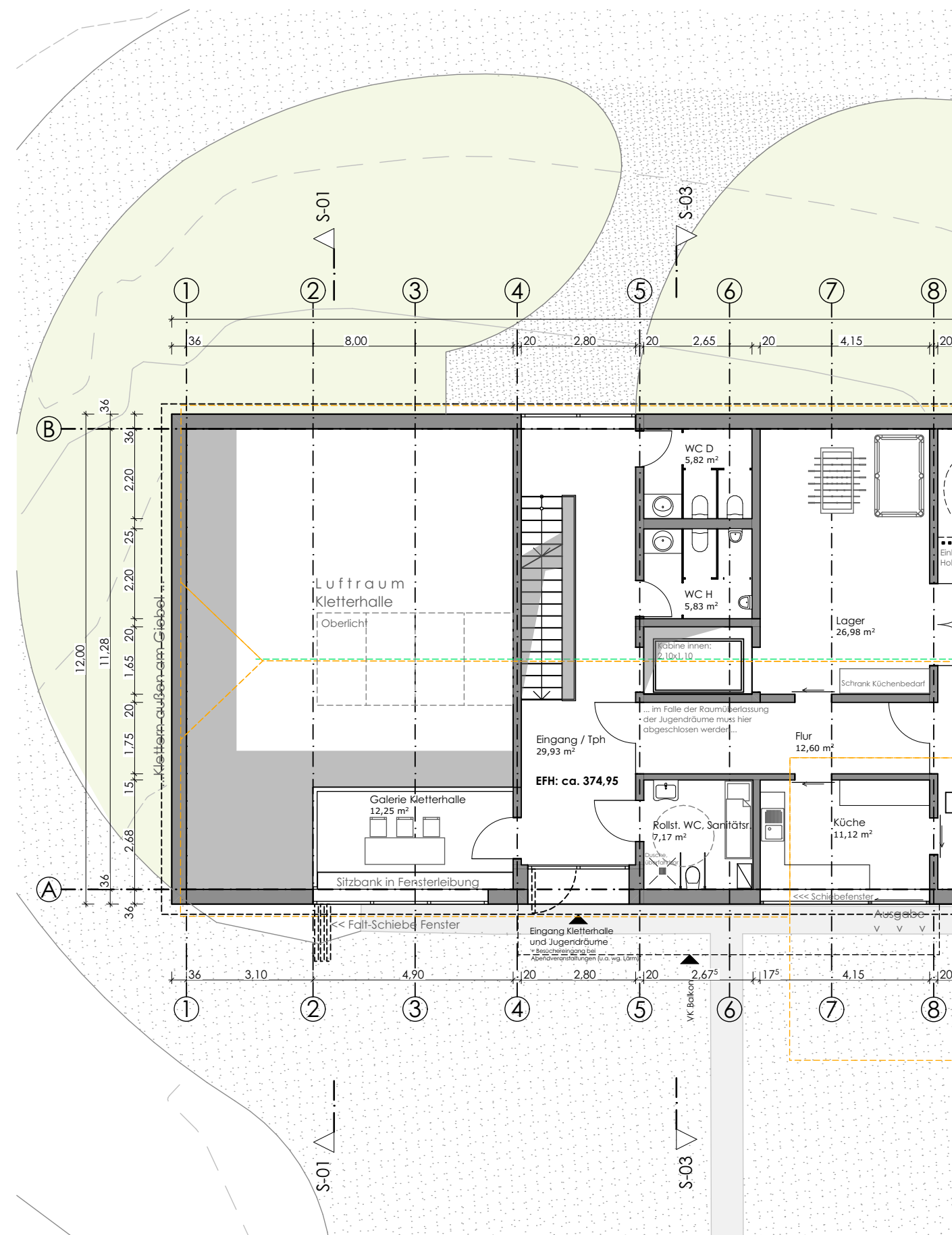
ERDGESCHOSS - Ausschnitt Kletterhalle
