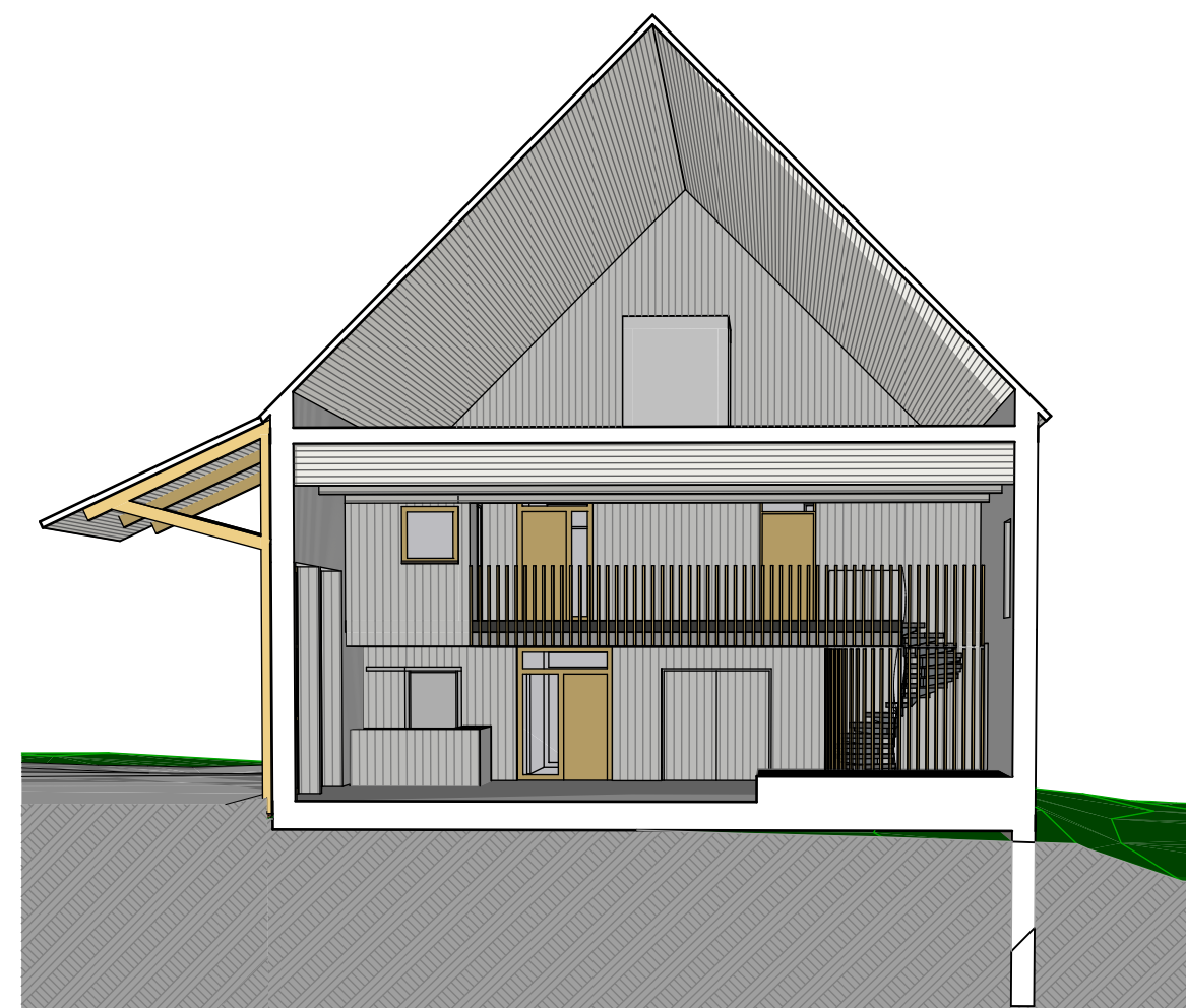
SCHNITT-PERSPEKTIVE MEHRZWECKRAUM
