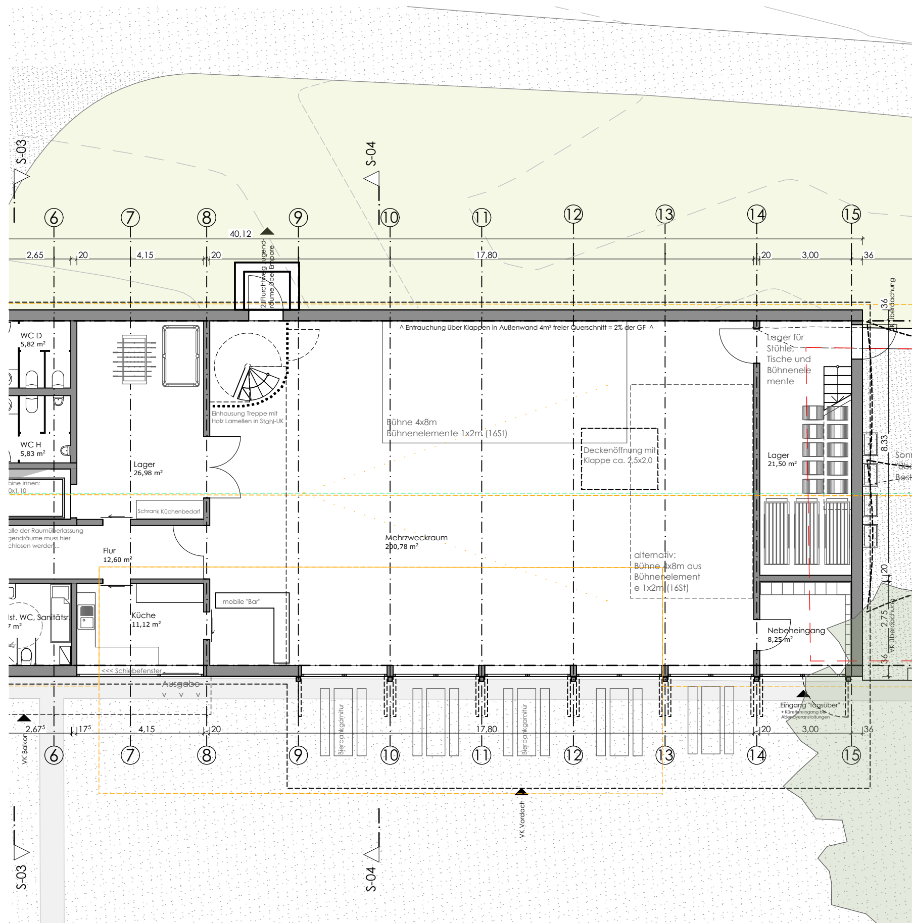
GRUNDRISS AUSSCHNITT - Mehrzweckraum
