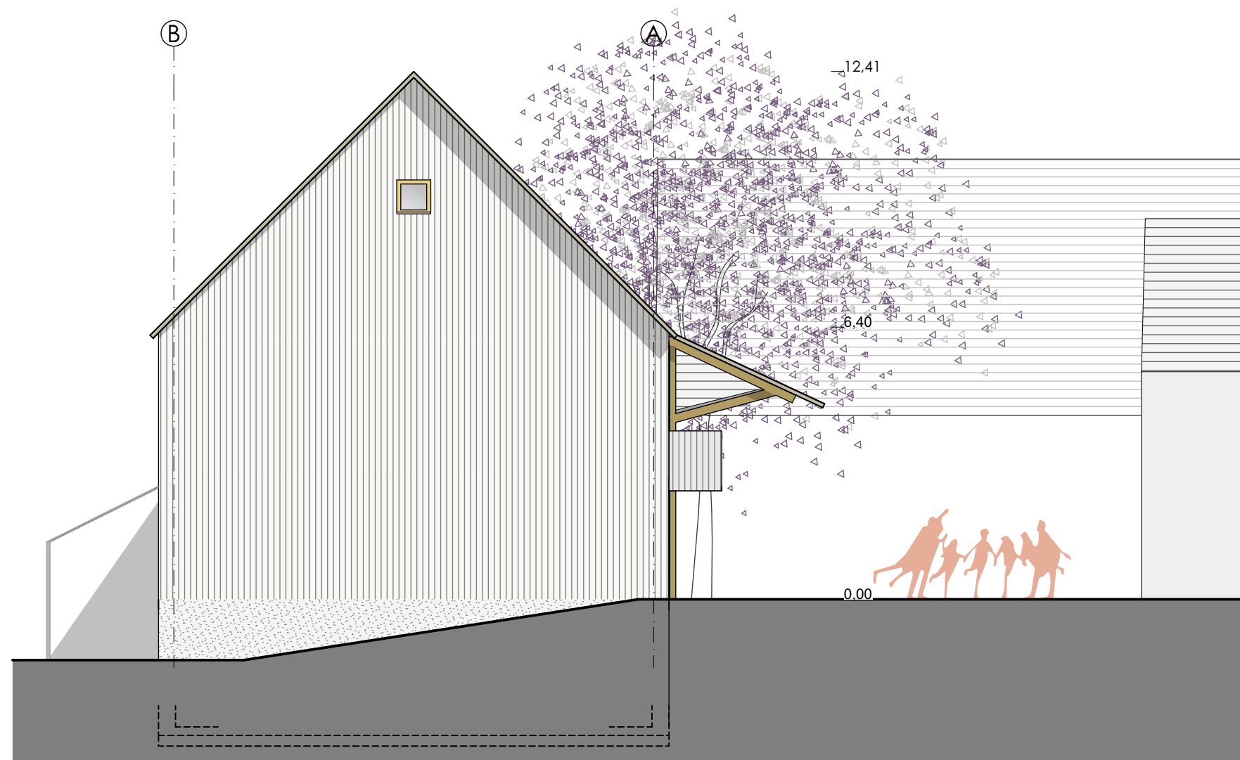
ANSICHT West
