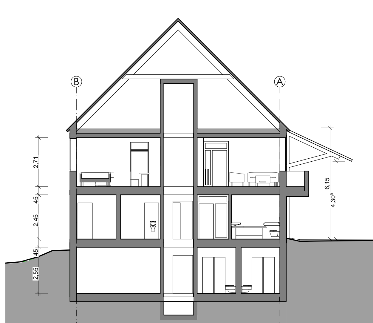
SCHNITT 1-1
